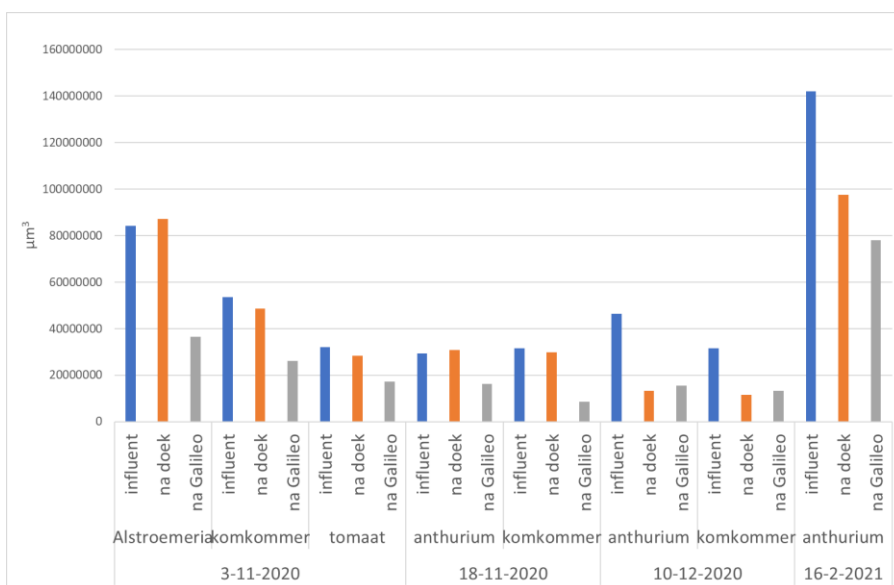
Figuur 3-23 Totaal volume aan deeltjes per mL in filterstraat 3
