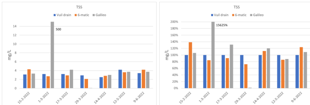
Figuur 3-34 TSS metingen op de verschillende momenten van monsternamen bij Verhoeven.
