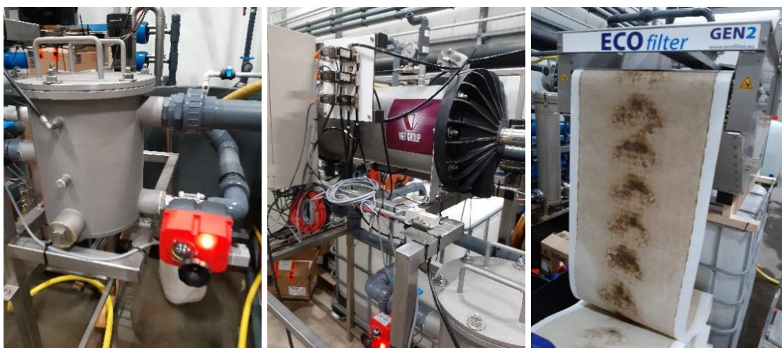
Figuur 2-5 Filterstraat bij Maarel Orchids. Van links naar rechts: gaasfilter ( Fiber Filtration ), MT-IBA filter ( Fiber Filtration ) en papierbandfilter ( Ecofilter ).
