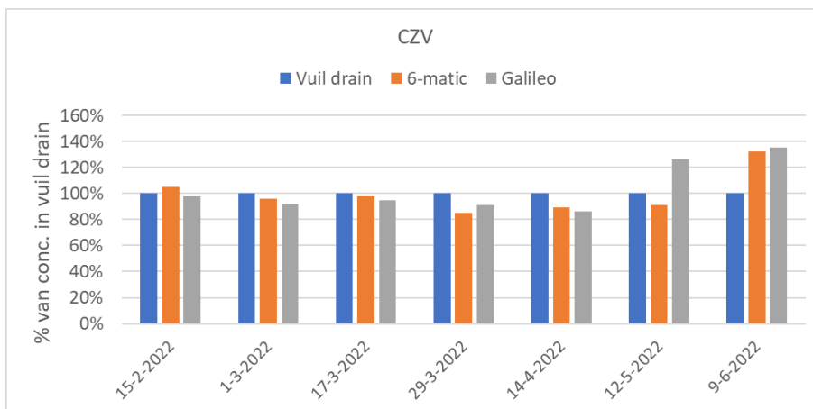
Figuur 3-35 CZV meting op de verschillende momenten van monsternamen bij Verhoeven.
