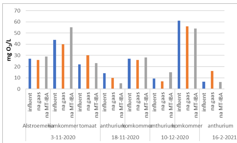
Figuur 3-16 CZV in filterstraat 1.
