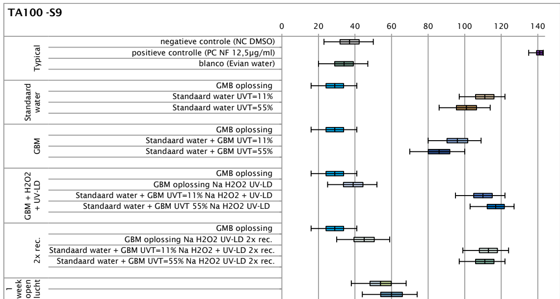
FIGUUR IV-3 RESULTATEN AMES FLUCTUATIE TEST BACTERIESTAM TA100 -S9
