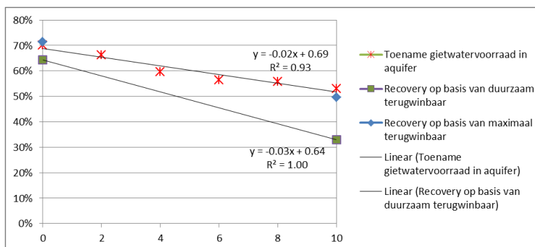
FIGUUR B2.1 VERLOOP VAN DE OMVANG VAN DE ZOETWATERBEL NA INJECTIE VAN ADDITIONEEL INJECTIEWATER. OP DE Y-AS IS DE ADDITIONELE OMVANG VAN DE ZOETWATERBEL WEERGEGEVEN RELATIEF T.O.V. DE HOEEVELEHID ADDITIONEEL GEINJECTEERD WATER. DE ADDITIONELE OMVANG IS HET VERSCHIL IN OMVANG VAN DE ZOETWATERBEL BEREKEND MET EN ZONDER EXTRA INJECTIE.
